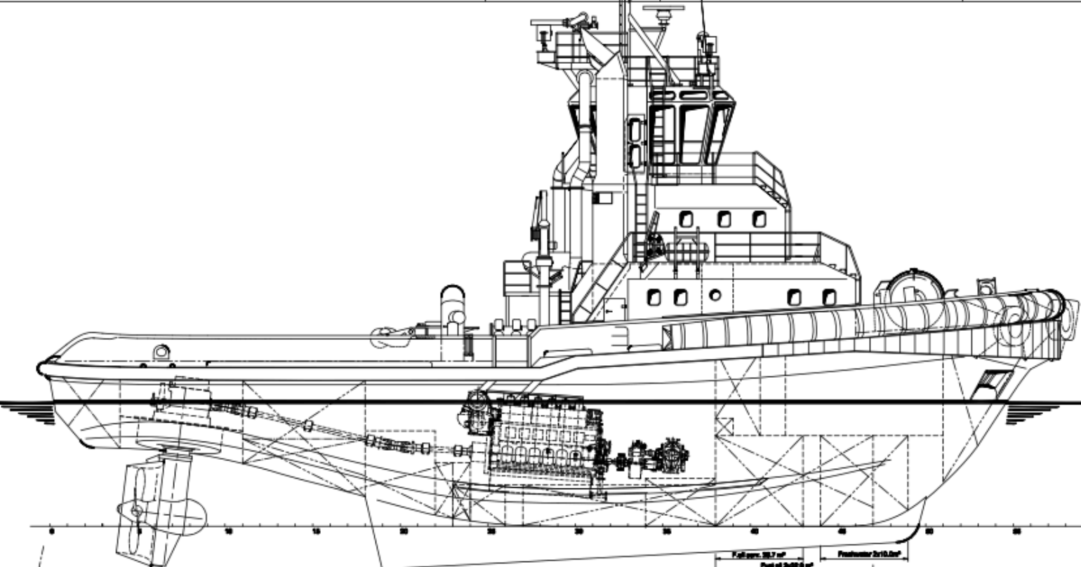
Maindeck
